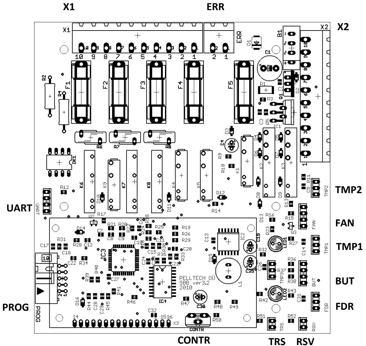
Рисунок 11 Плата контроллера
