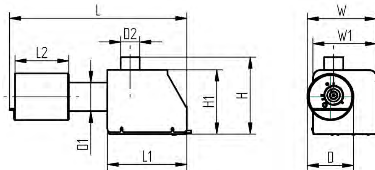
Рисунок 2 Размеры
